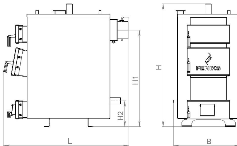
Рисунок 1 – Позначення габаритів котла
