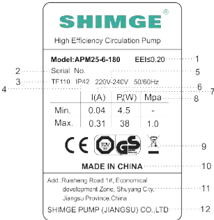
Рисунок 7. Заводська табличка
